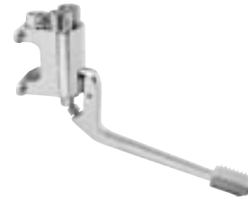
Miscelatore monopedale a parete H51GFS08 [LxPxH] 86x275x200 mm
