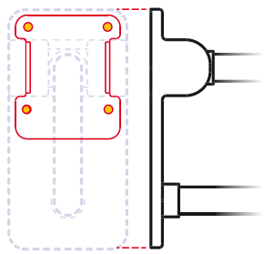
Acciaio inox - AISI 304 122x145 [LxH] mm
